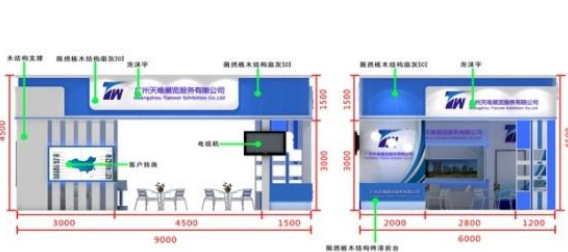
正面立面图
