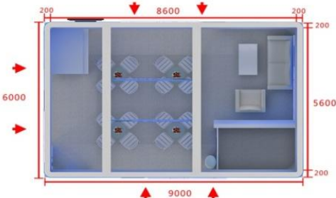
平面布置图
