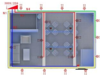
电气平面布置图
